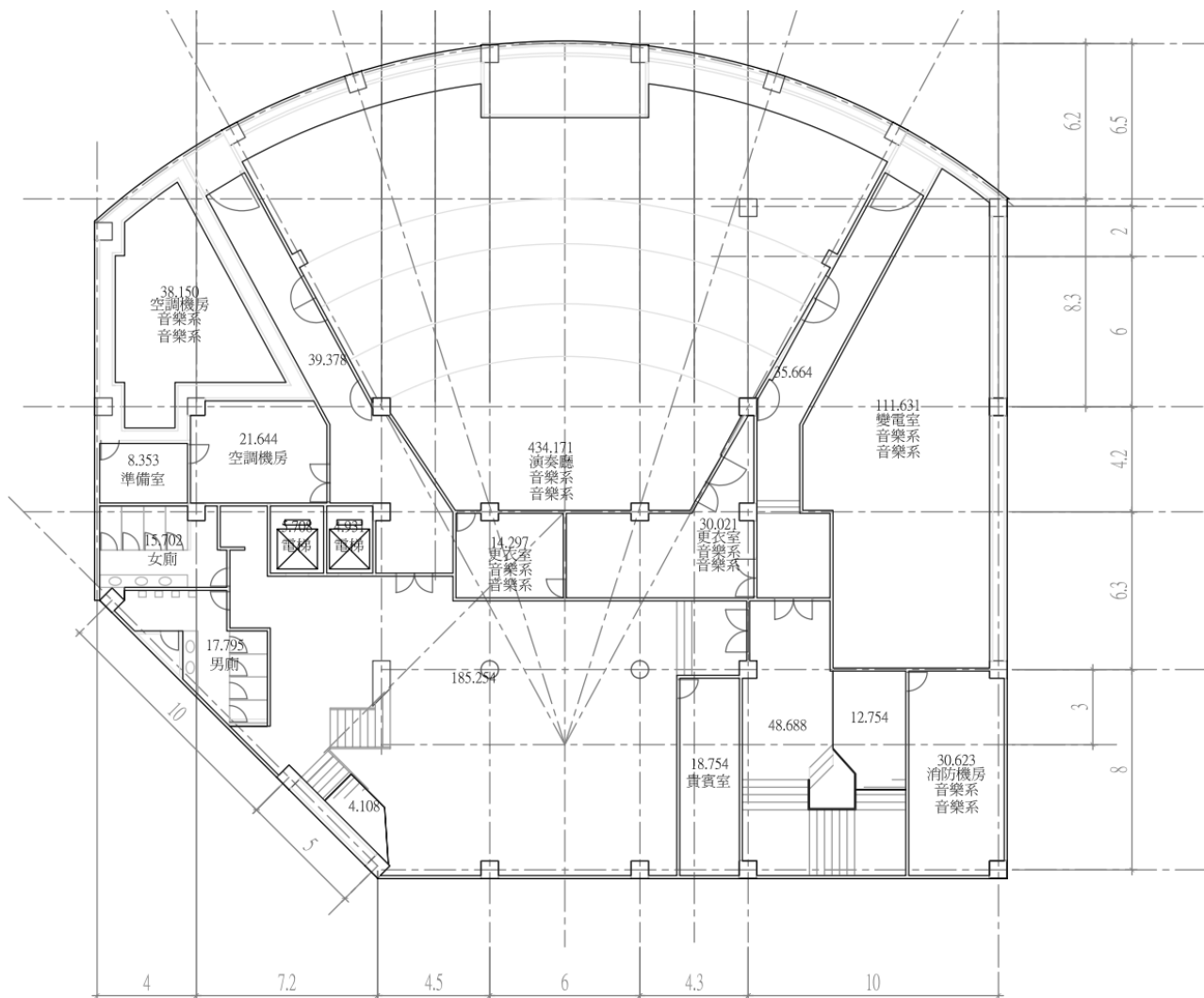
藝術學院地下層平面
