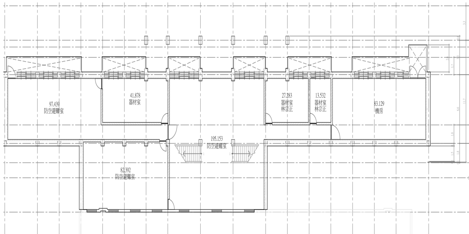
游泳池看台地下層平面
