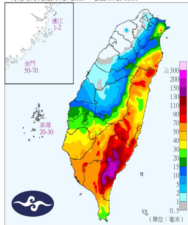
定量降水預報 (Ⅳ)
