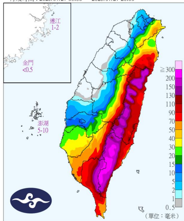
定量降水預報 (Ⅲ)
