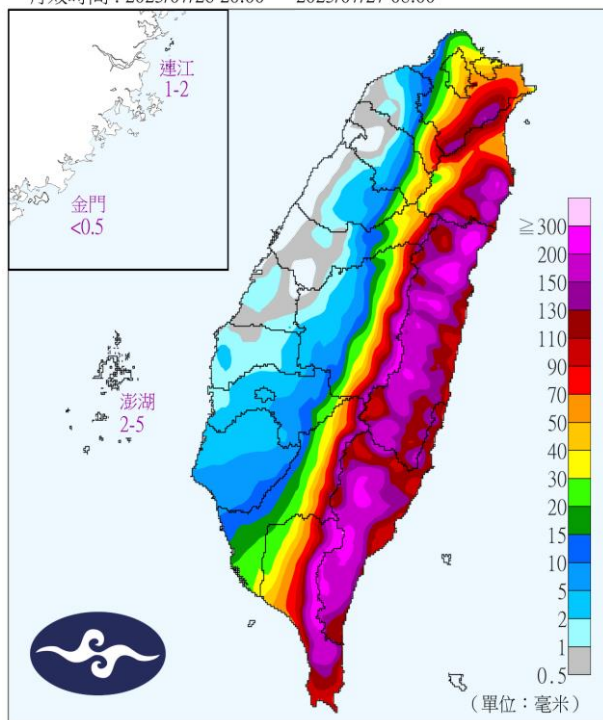
定量降水預報 (Ⅱ)
