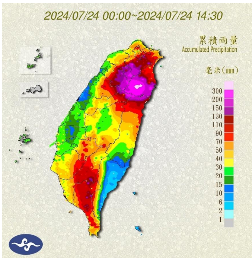
累積雨量
