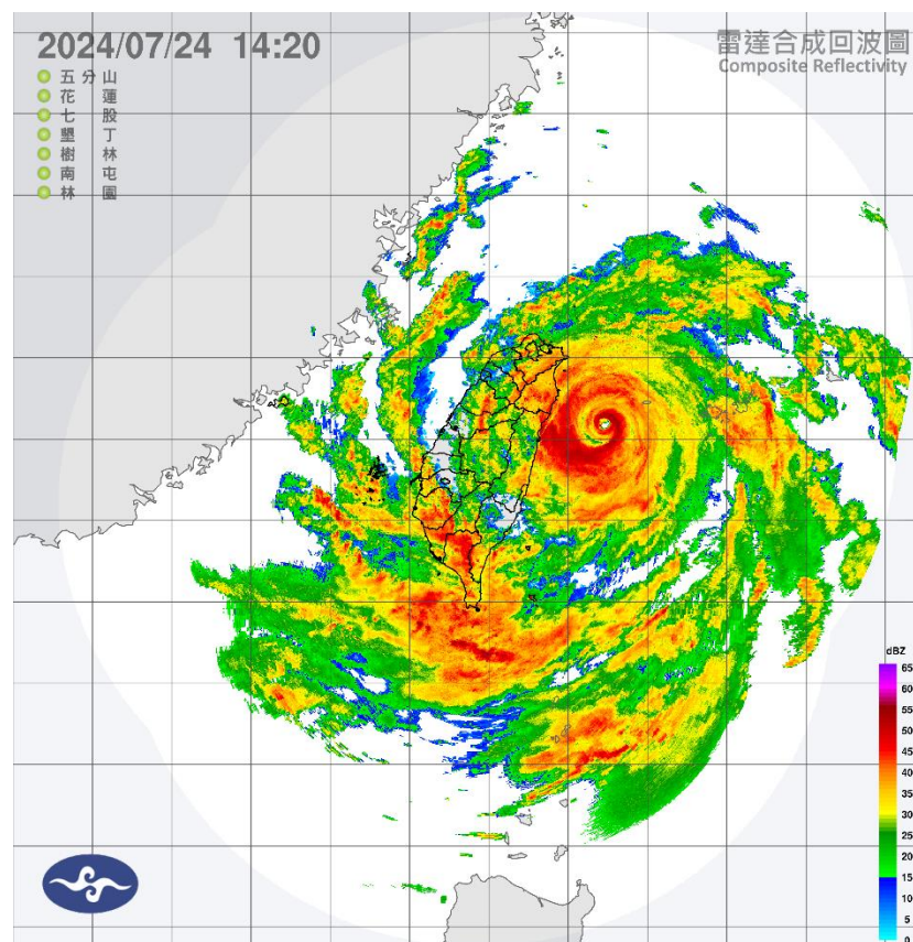
雷達迴波圖
