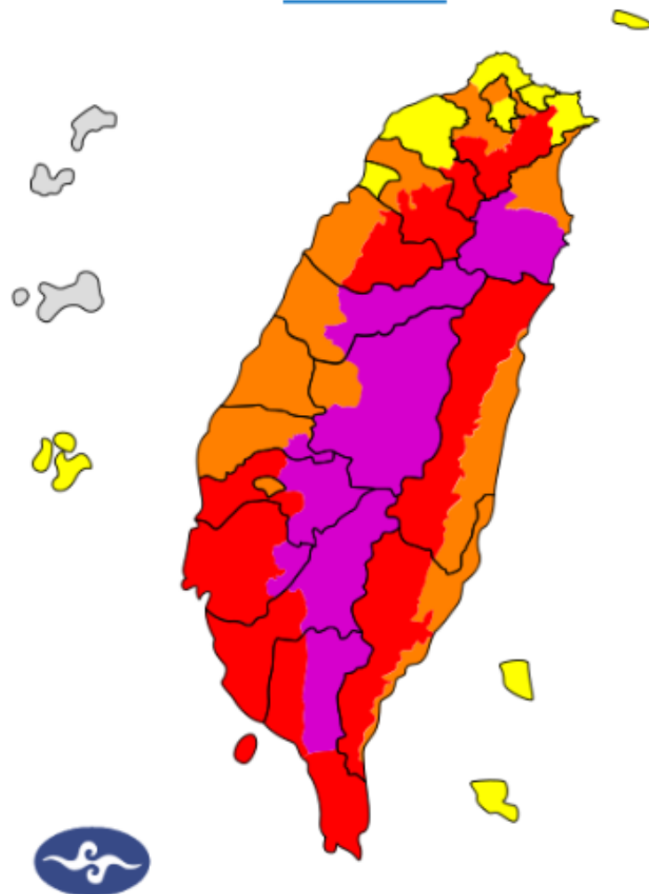
豪雨特報
