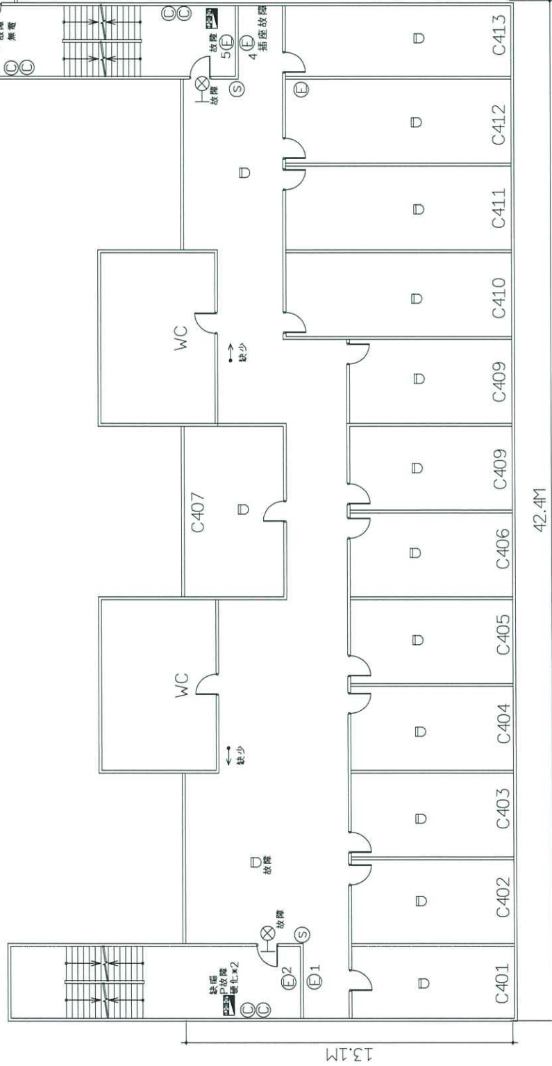
中山大學翠亨宿舍C棟4F消防設備平面圖
