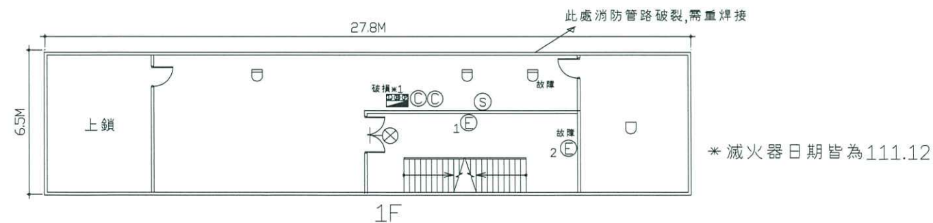
中山大學翠亨宿舍D棟宿舍消防設備平面圖
