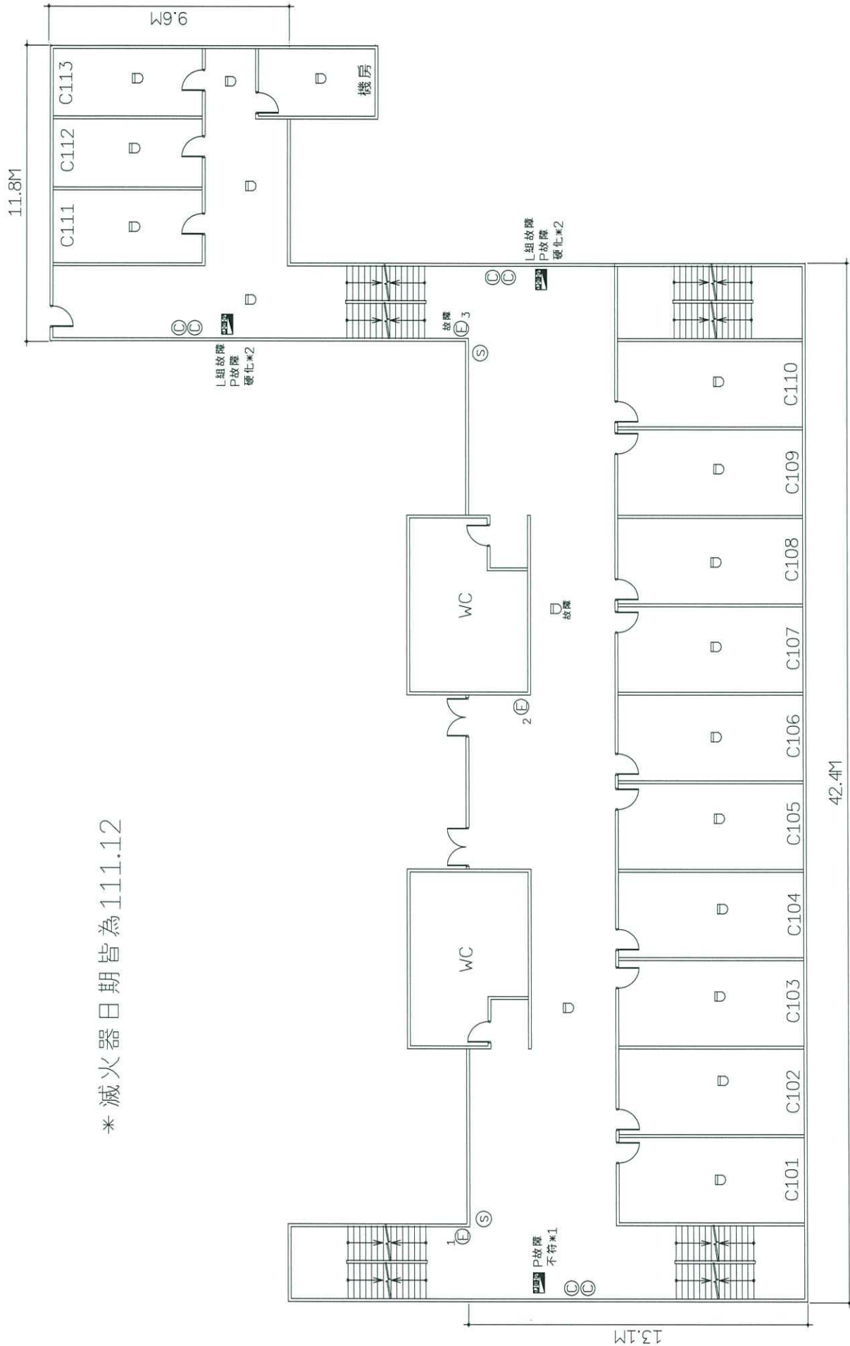
中山大學翠亨宿舍C棟1F消防設備平面圖
