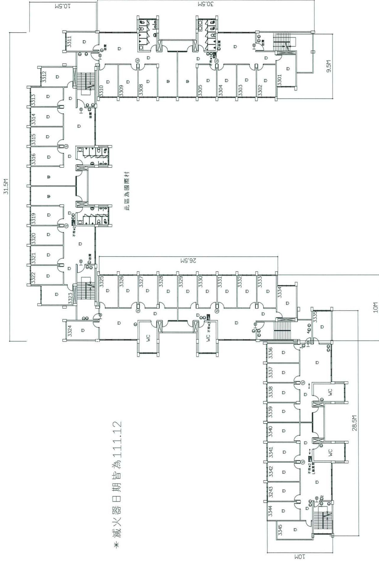
中山大學武嶺三村3F消防設備平面圖
