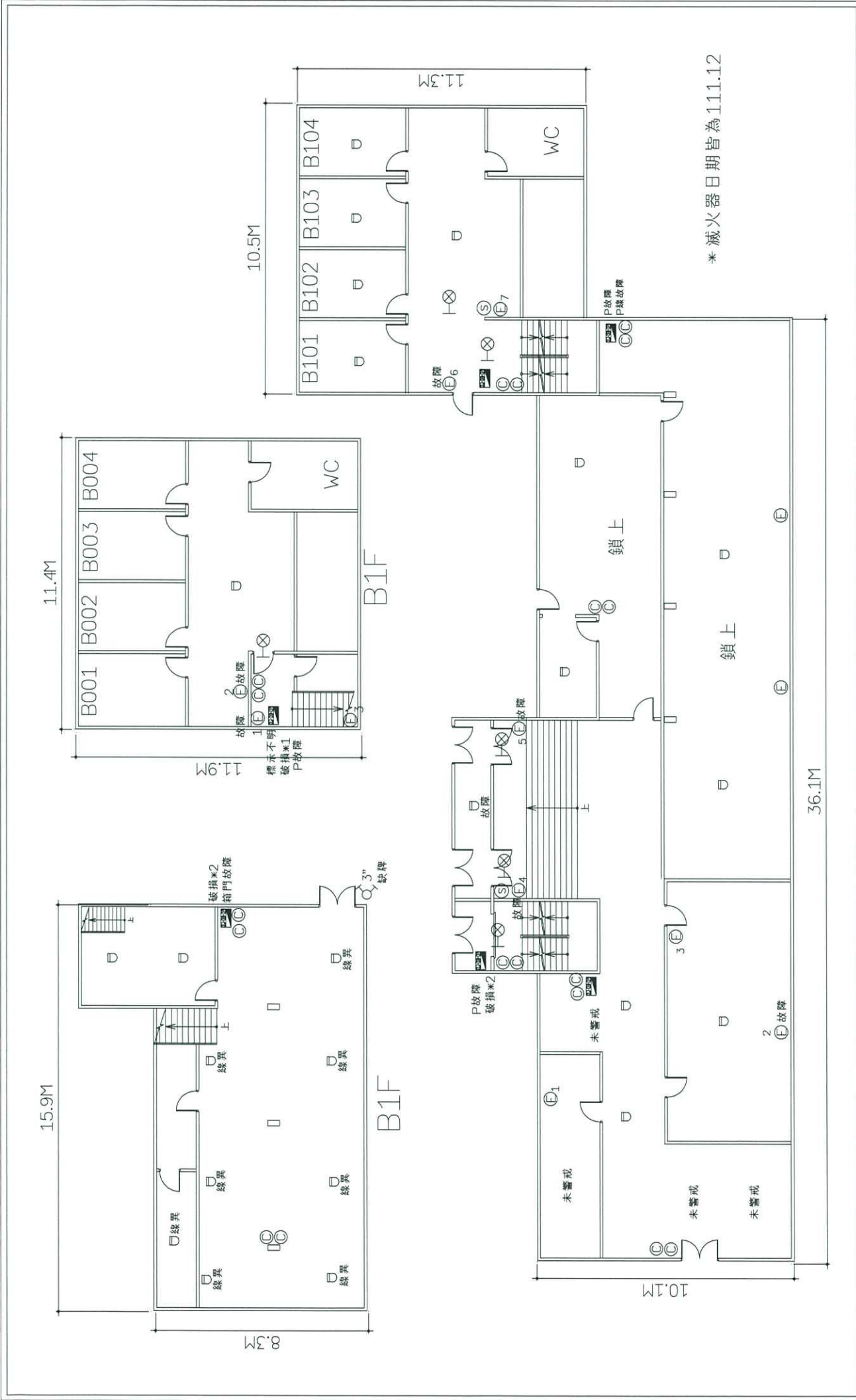
中山大學翠亨宿舍B棟1F消防設備平面圖
