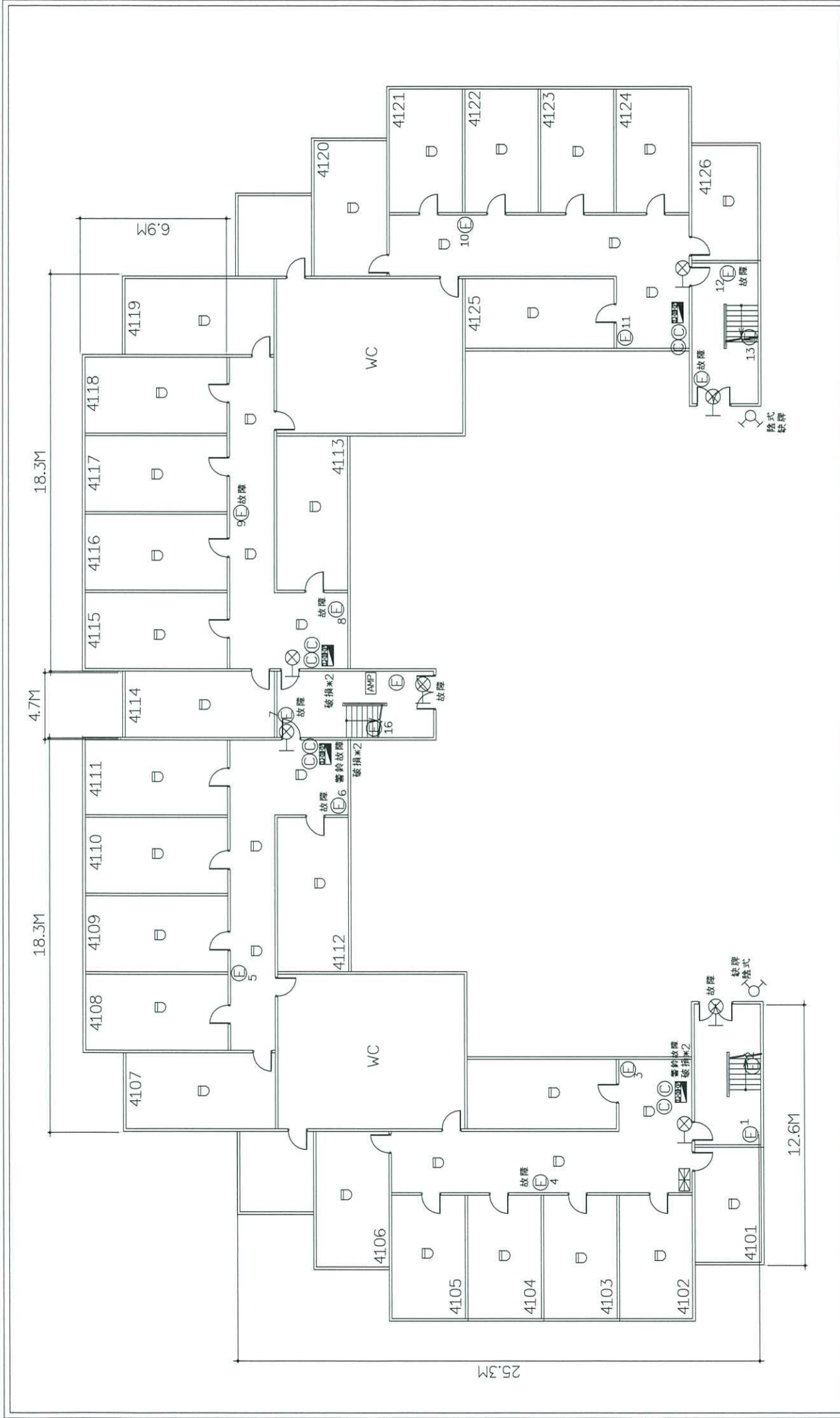
中山大學武嶺四村1F消防設備平面圖
