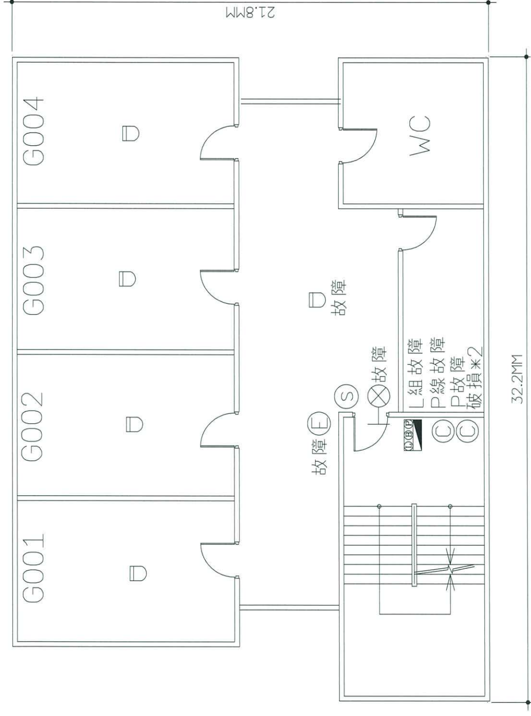
中山大學翠亨宿舍G棟B1F消防設備平面圖
